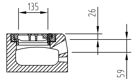
Schnitt A-A
