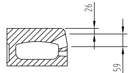
Schnitt A-A
