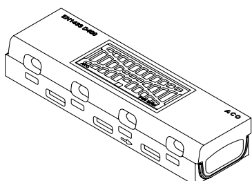
KerbDrain Bridge Inspektionselement (OPA)
