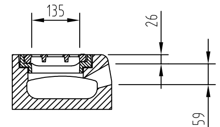
Schnitt A-A
