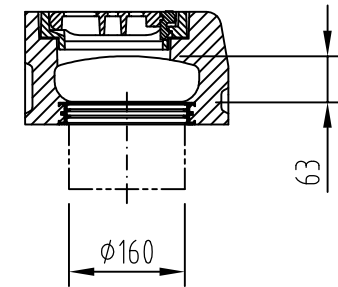
Schnitt A-A
