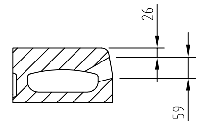
Schnitt A-A
